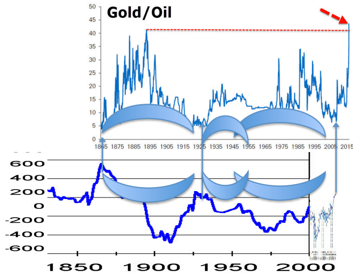
Соотношение цены золото/нефть и скорость вращения Земли (LOD) в XIX – XX веках со сдвигом на 7 лет
