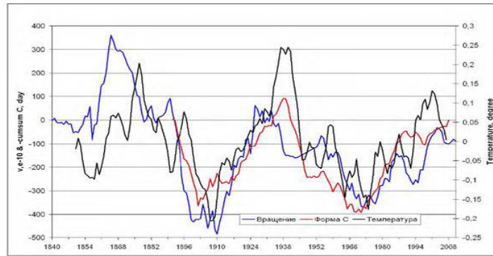
Синхронные изменения скорости вращения Земли ( v \times 10^{10} ) в относительных единицах (сплошная синяя), накопленных аномалий годового числа дней с процессами формы циркуляции -С (красная) и скользящих средних за пять лет глобальных аномалий температуры воздуха после исключения тренда по данным HadCRUT3 (черная).
