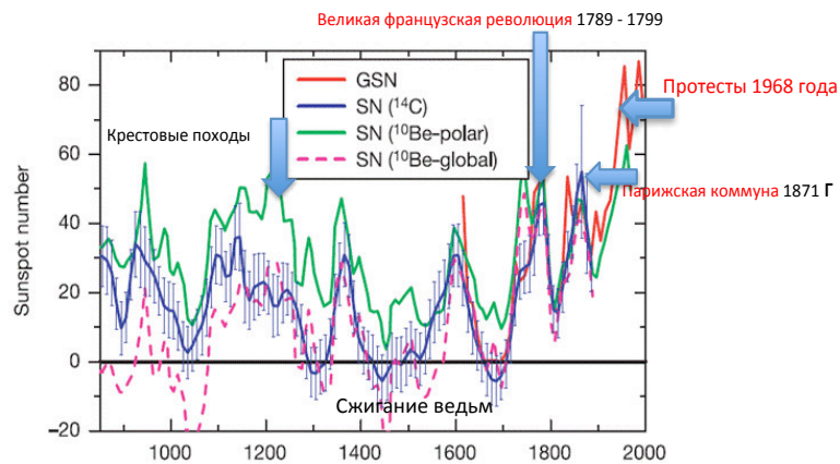
Рисунок. Сопоставление количества солнечных пятен (GSN), содержания изотопов ^{14}\text{C} в древесине и ^{10}\text{Be} в полярных льдах для периода 850-2000 годов
