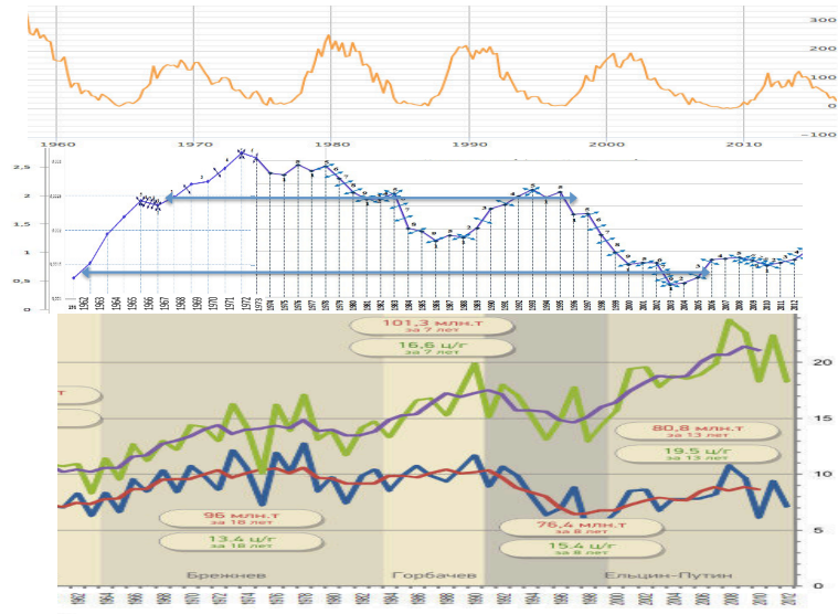
Число Вольфа , LOD Земли и урожайность пшеницы в России с 1962 года
