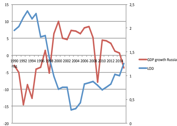
Темпы роста ВВП в России и изменение LOD Земли
