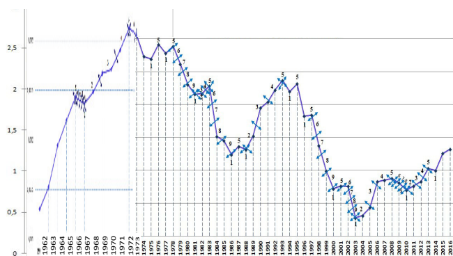
Данные по LOD Земли с 1962 года в мс.
