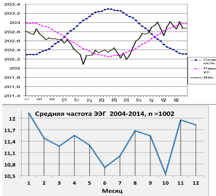
Графики изменения скорости движения Земли по орбите и средней частоты ЭЭГ
