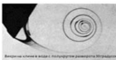
Вихри на клине в воде с полусферой радиуса 30 градусов
