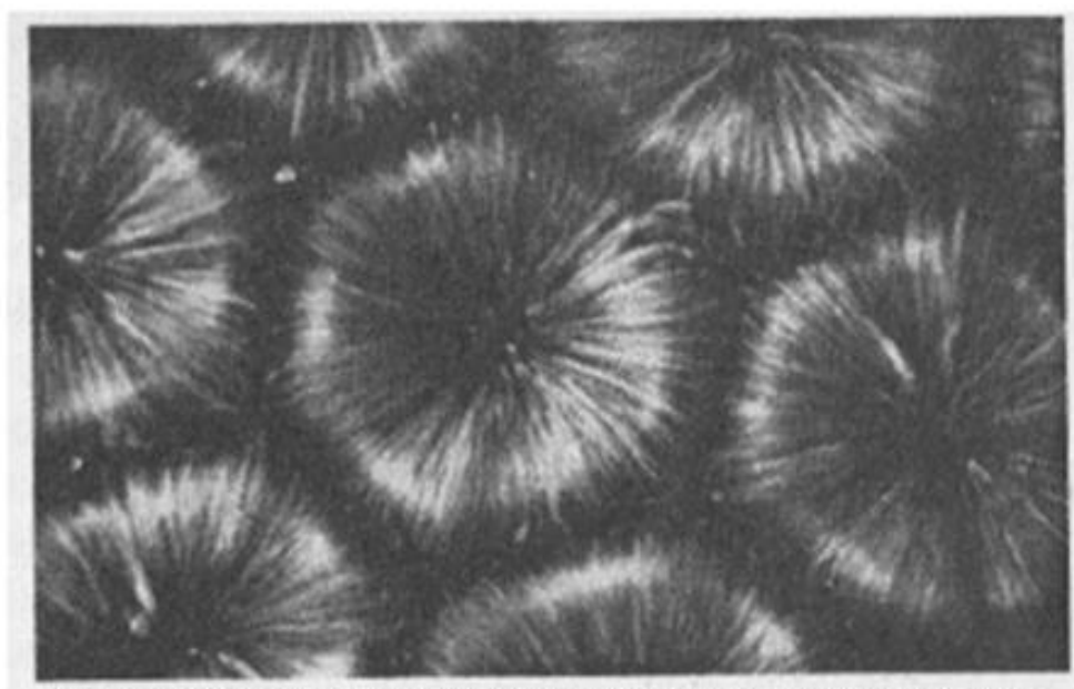
Фотография слоя силиконового масла глубиной 1 мм при равномерном нагреве снизу. Свет, отраженный от алюминиевых хлопьев, демонстрирует подъем жидкости в центре каждой ячейки и ее опускание на краях
