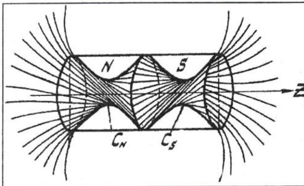
Поле постоянного магнита (И.Ф. Попов)
