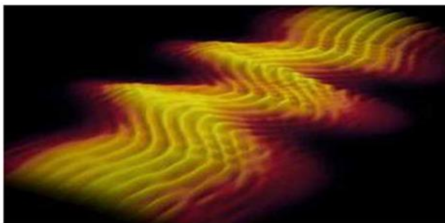
Фотография световой волны.
