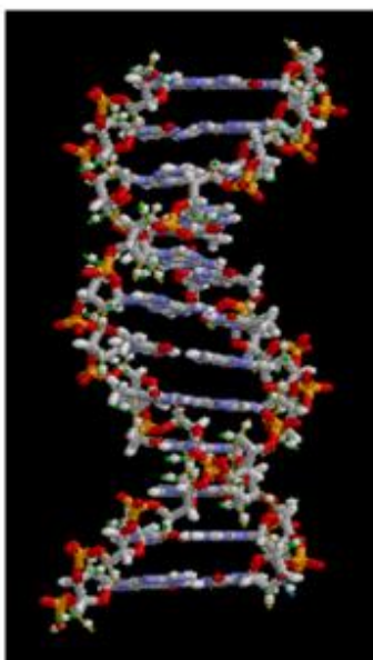
Структура двойной спирали ДНК. Атомы в структуре имеют цветовую кодировку элемента
