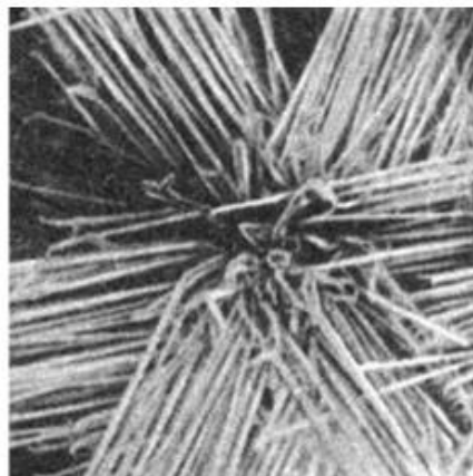
Нитевидные кристаллы AlN (электронно-микроскопич. изображение, увеличено в 3000 раз).
