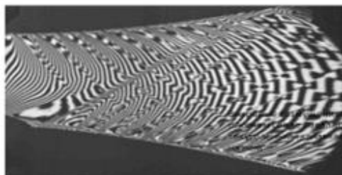
Вихревые возмущения в плоском сопле Лавала с трехугольными канавками на нем
